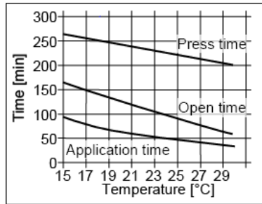
Диagr. 1 Время нанесения, время под прессом, время затвердевания для SikaForce®-7710 L100
